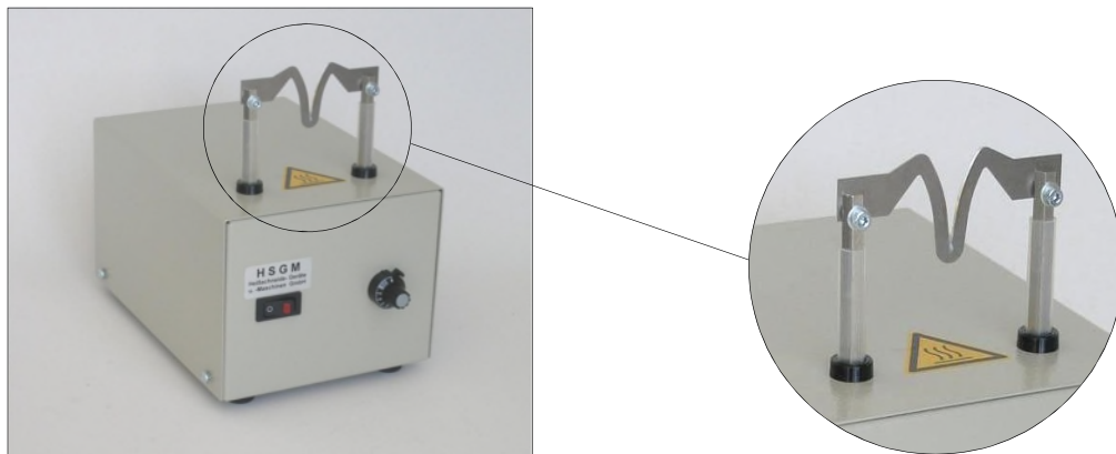
Foto zeigt Gerät HSG-00-VW mit eingesetzter Schneide HS-S-15°-60°-00-VW.
